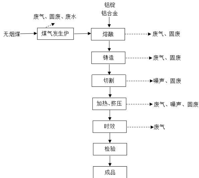
图3-2 环评设计中的原有生产工艺流程图
