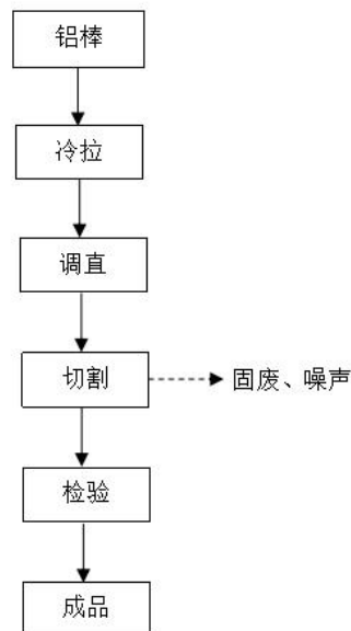
图3-4 实际建设的原有生产工艺流程图
