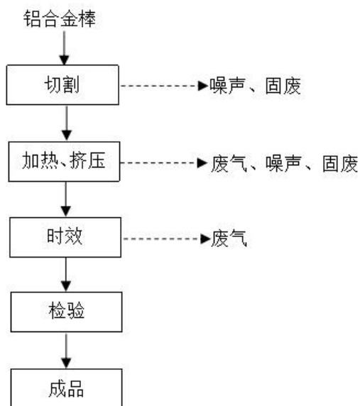
图 2-1 项目实际生产工艺
