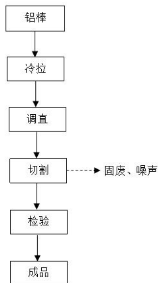
图3-2 环评设计中的原有生产工艺流程图
