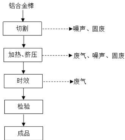
图3-4 实际建设的原有生产工艺流程图
